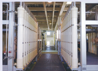
浄水施設の膜モジュール Membrane modules at a water purification plant
