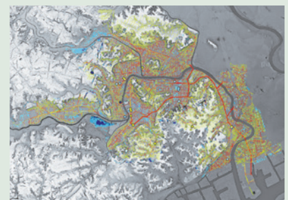
鶴見川低平地における河川と下水管内水位を統合的に解析する新たな都市浸水モデル A new urban inundation model that comprehensively analyzes water levels in river and drainage systems in the Tsurumi River lowland
